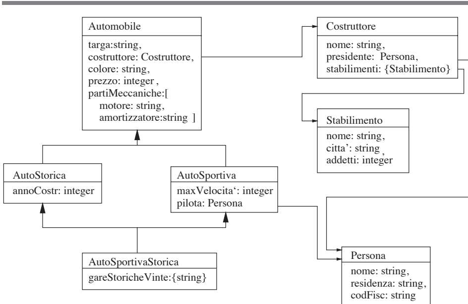
Figura 19.2 Schema di una base di dati a oggetti per la descrizione di automobili.
