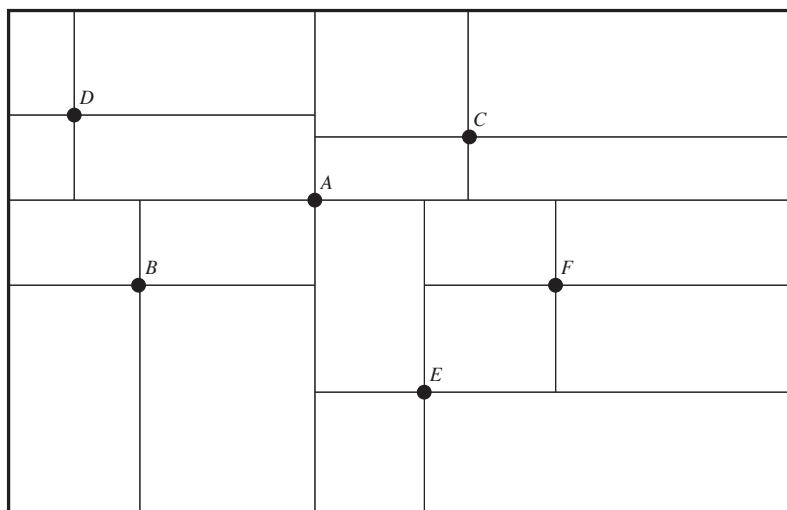
Figura 19.5 Un quad-tree.
