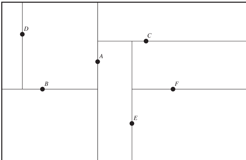
Figura 19.4 Un 2-d tree.
