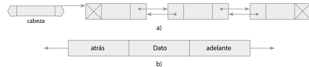
Figura 34.5 Lista doblemente enlazada. a) Lista con tres nodos; b) nodo.
