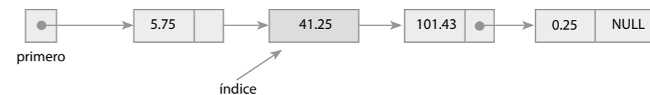
Figura 34.4 Búsqueda en una lista.
