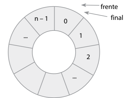
Figura 34.15 Cola con un elemento en un arreglo circular.
