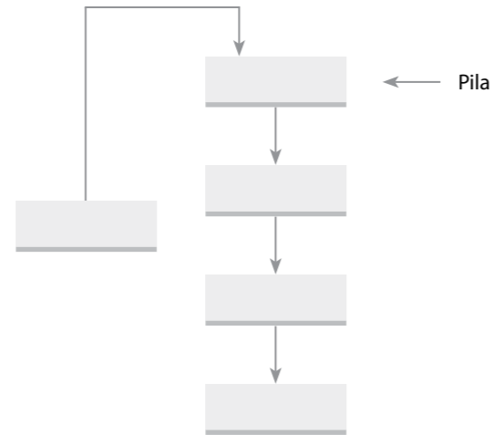
Figura 34.10 Representación de una pila con una lista enlazada.
